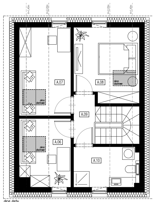
RZUT PODDASZA
